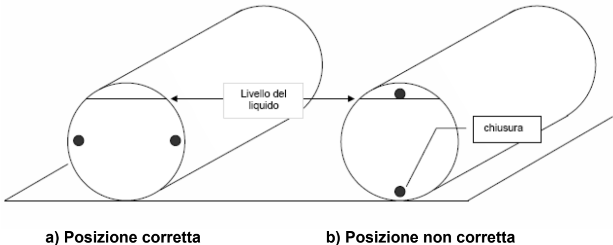
Figura 1 Imballaggi con chiusure munite di sfiato.
