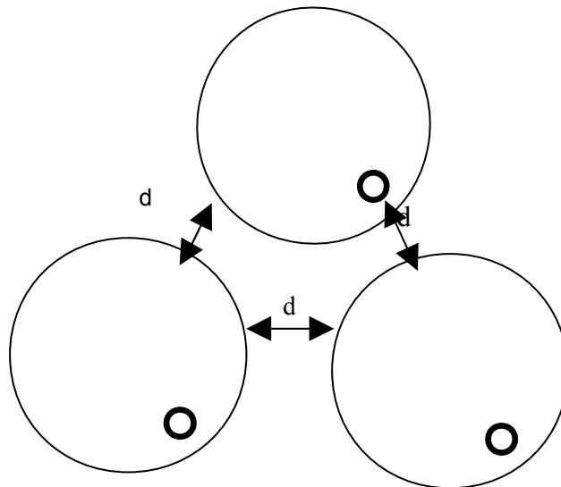
Figura 3 Vista in pianta dei fusti
